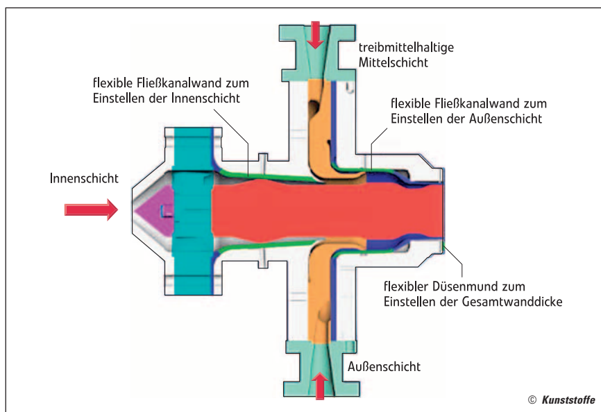
Bild 5. Das in der Querschnittsdarstellung gezeigte Dreikanalrohrwerkzeug mit drei flexiblen Wandbereichen ist sehr kompakt gebaut und besteht nur aus acht Einzelteilen
