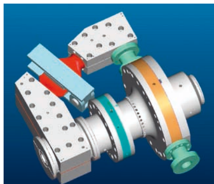
Bild 8. Dreidimensionale Darstellung des kompletten Dreikanalrohrwerkzeugs mit der im Anströmkanal für die Deckschicht integrierten Drossel (rot)
