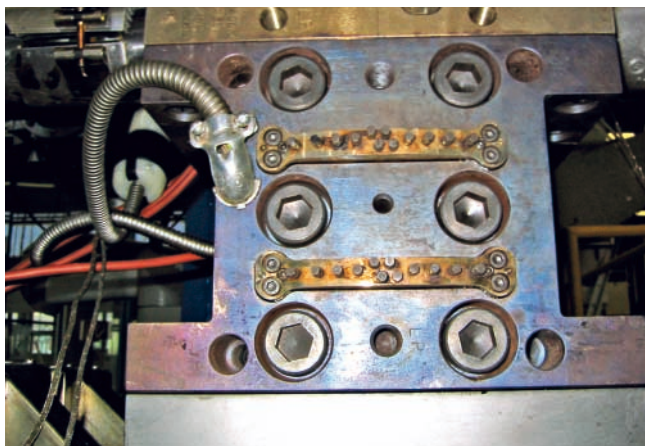
Bild 2. In eine Technikumsanlage eingebauter 3-Kanal-Membranadapter, mit dem sich am Zusammenströmpunkt die Geometrie des 50 mm breiten Fließkanals jeweils mit 12 Stellschrauben feinfühlig optimieren lässt (alle Bilder außer Bild 1: Groß Kunststoff-Verfahrenstechnik)
