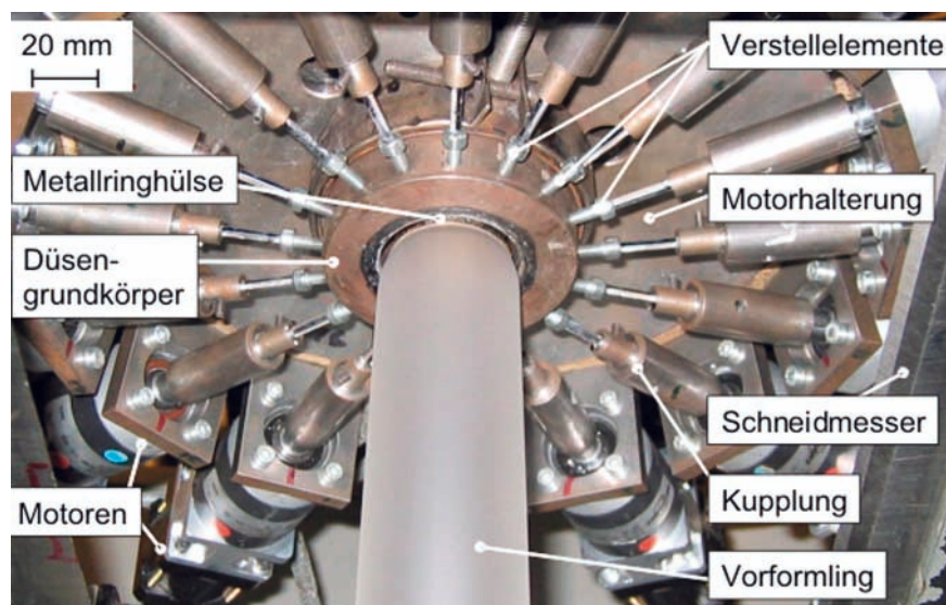
Bild 1. In eine Blasformanlage eingebautes Flexringwerkzeug mit einem Durchmesser von 35 mm, das mit 16 Stellantrieben dynamisch verstellt werden kann (Foto: IKV)
