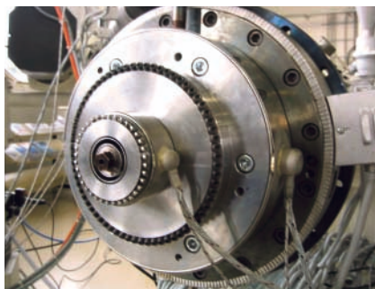
Bild 3. Zweikanalwerkzeug mit einer integrierten Flexringhülse zur Feineinstellung der Schichtdicke der Deckschicht (hintere Stellschrauben) sowie der Gesamtdicke (Stellschrauben am Düsenmund)
