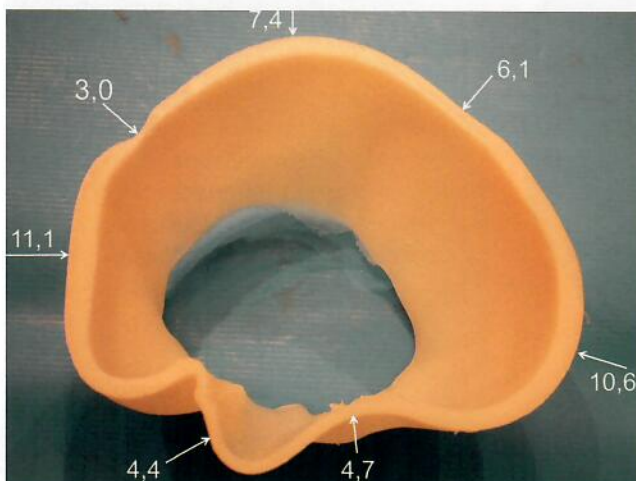
Bild 6: Erforderliche Wanddickenverteilung, um das Teil auch im Blasformverfahren aufblasen zu können
