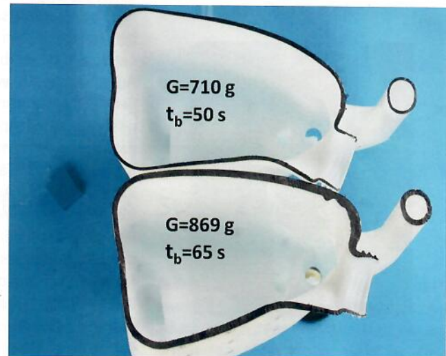
Bild 1: Resultierende Wanddickenverteilung, das Gewicht und die Zykluszeit die mit einer GWDS-Düse erreicht worden ist
