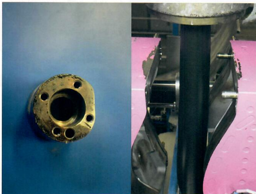
Bild 4: Links, Dornprofilierung für den Scheibenwaschwasserbehälter; rechts, gerader, wellenfreier Vorformling zur Herstellung des Behälters
