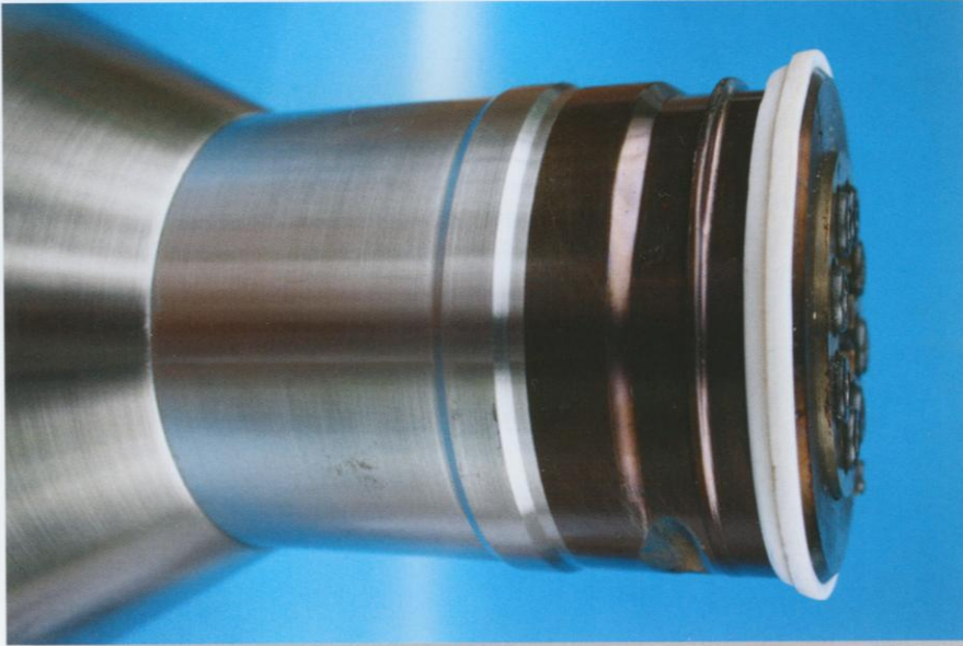
Bild 5: 3D Dorn, mit dem der Kraftstoffkanister in Bild 4 hergestellt wurde (Werkbilder: Dr. Ing. Heinz Groß, Kunststoff-Verfahrenstechnik, Roßdorf)
