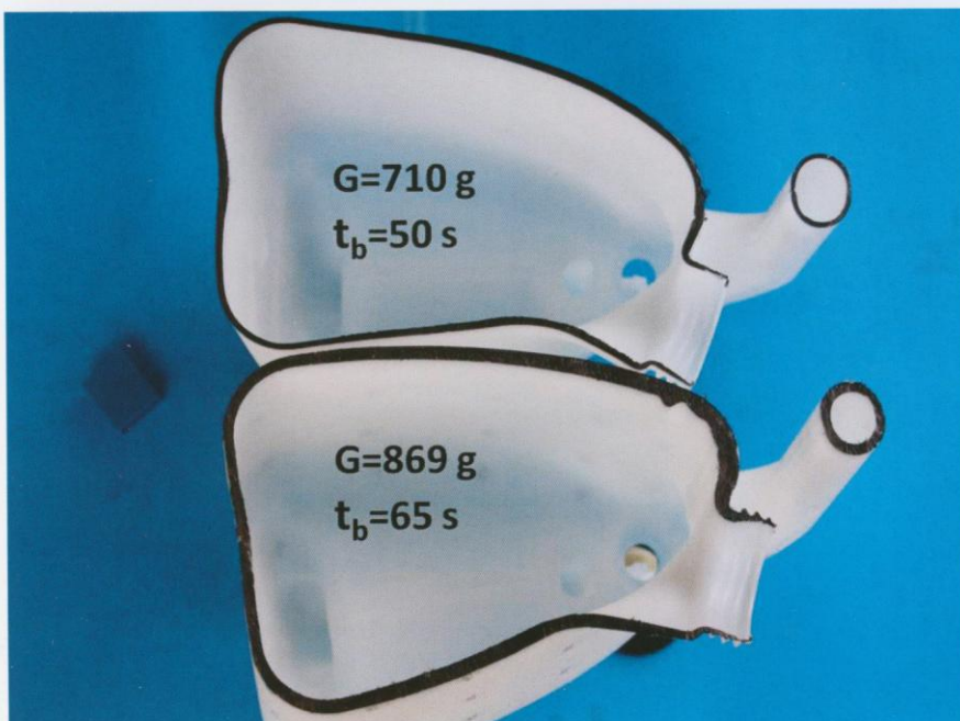
Bild 4: Kanister, hergestellt mit konventioneller Technik (unten) und 3D Technik (oben) G = Gewicht, t_b = Blaszeit
